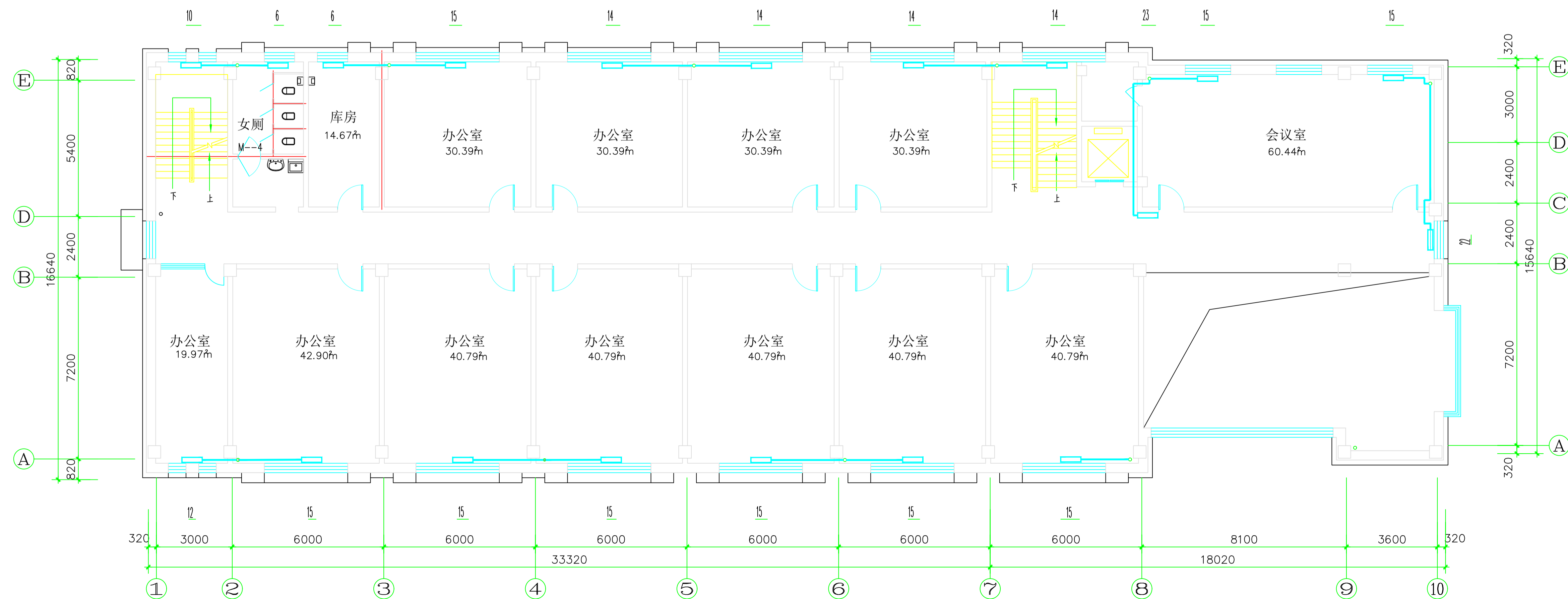
二层供暖平面图 1:100
