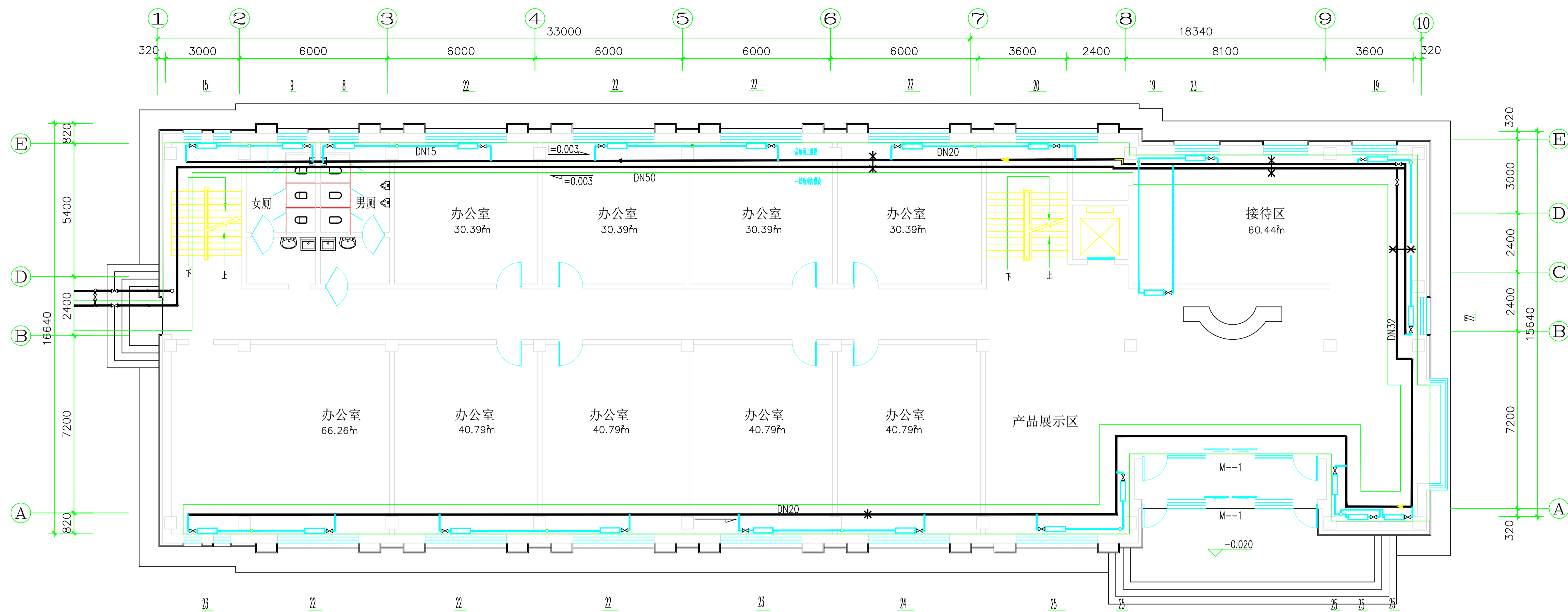
一层供暖平面图 1:100
