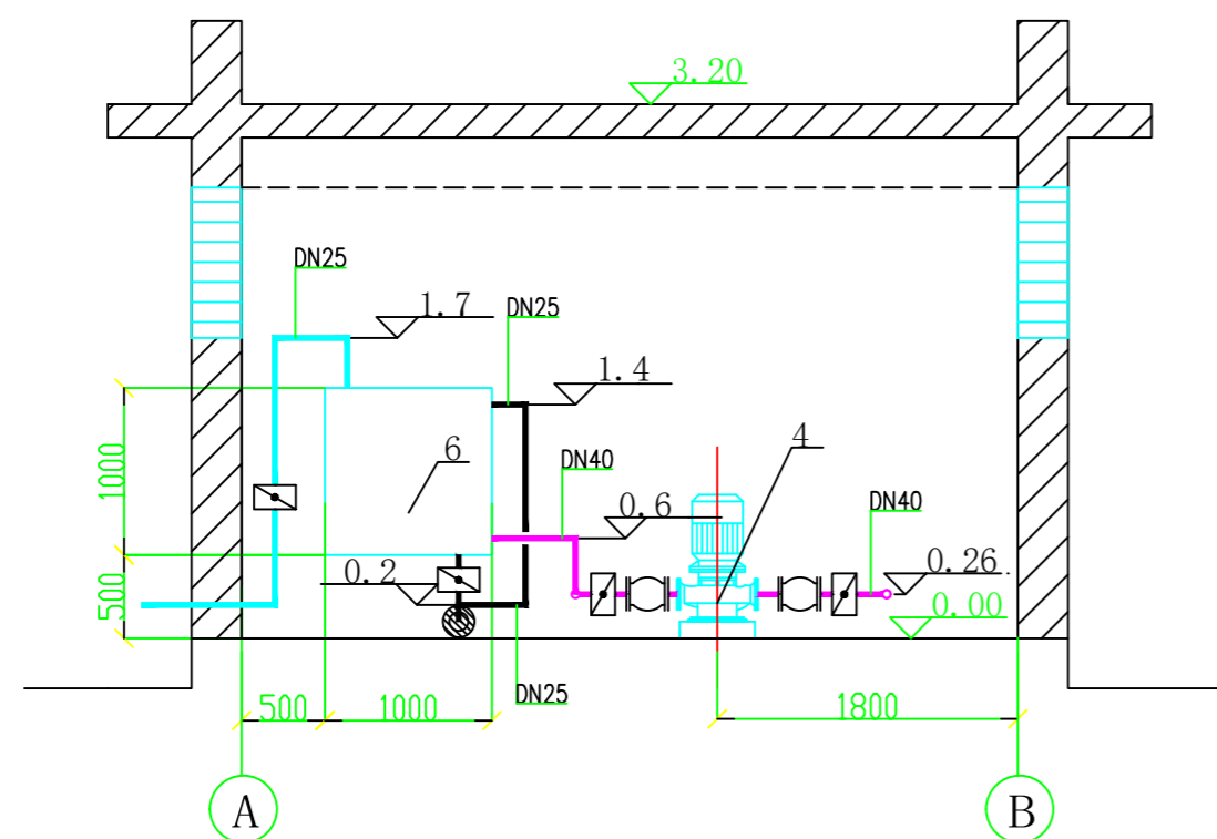
A-A剖面图 1:50
