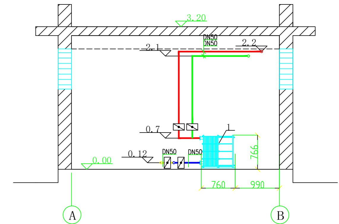
C-C剖面图 1:50
