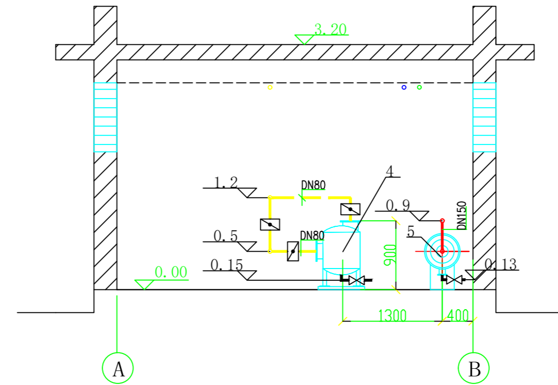
B-B剖面图 1:50
