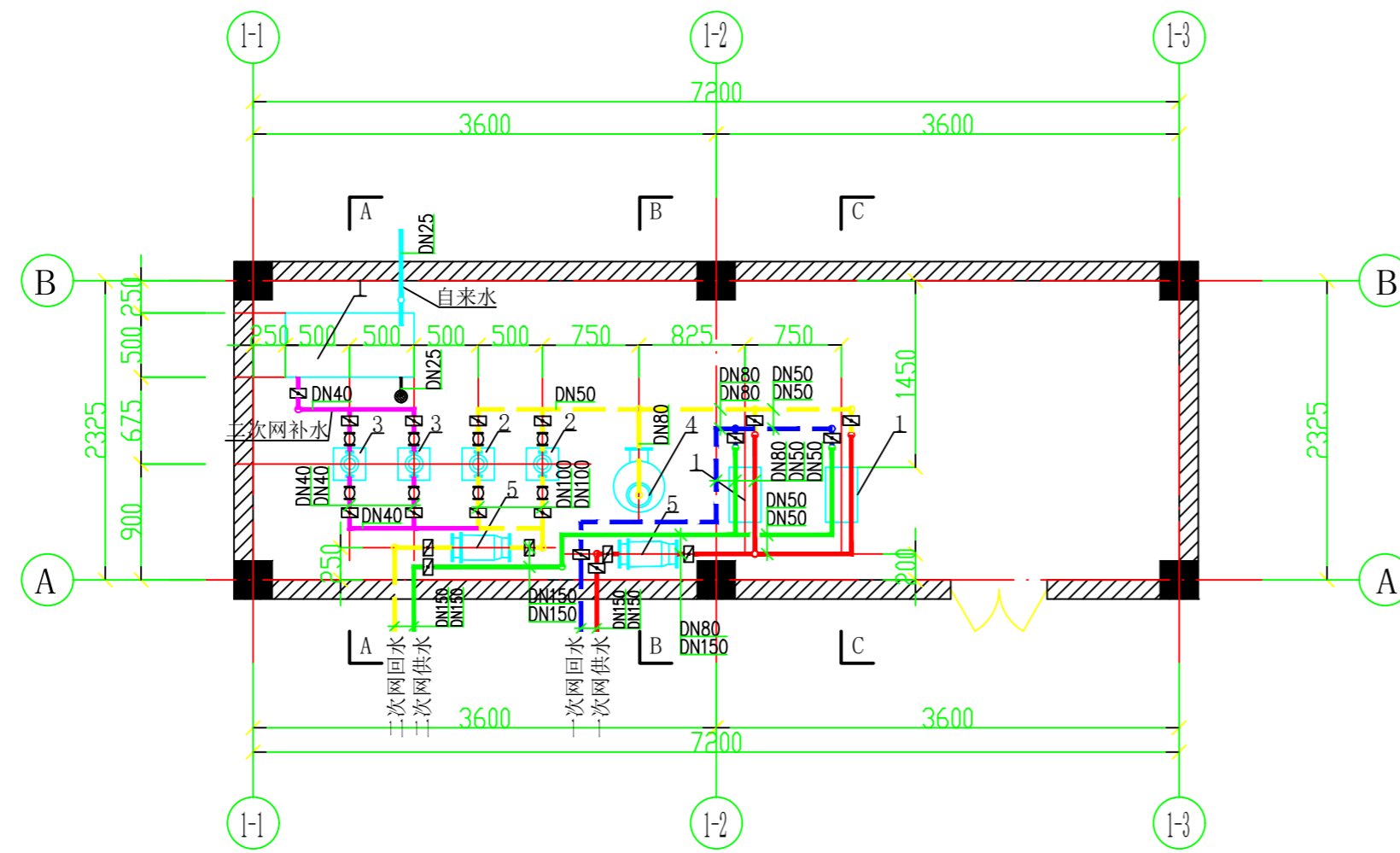
换热站设备、管道平面图 1:100
