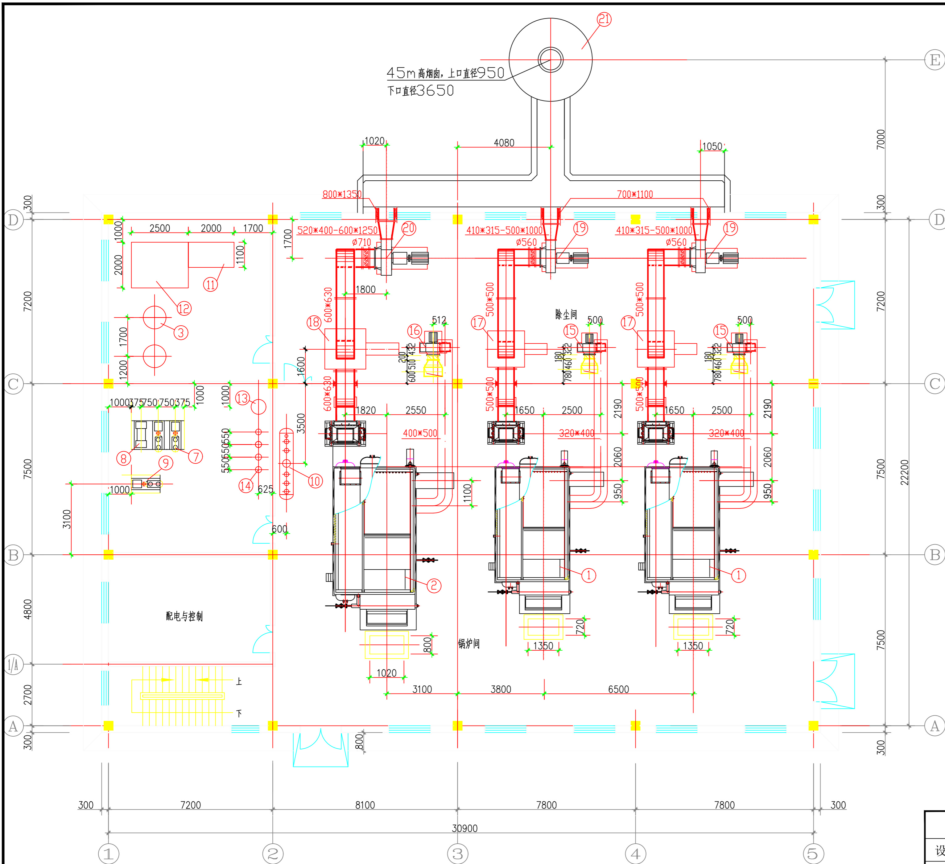
一层锅炉房设备平面布置图 1:100
