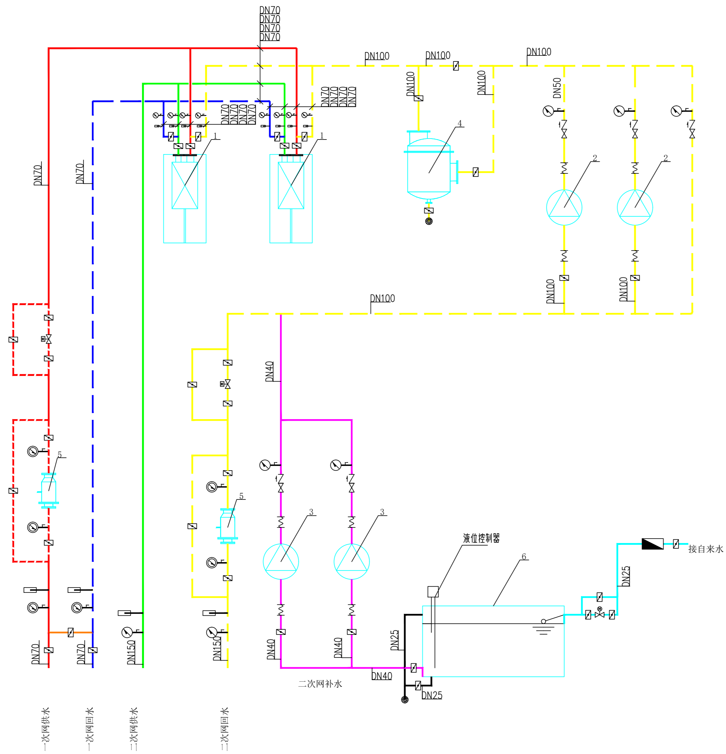
热力系统图
